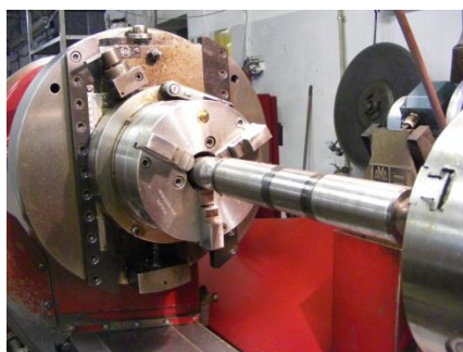
Szlifowanie wałka na szlifierce AMC-Schou
