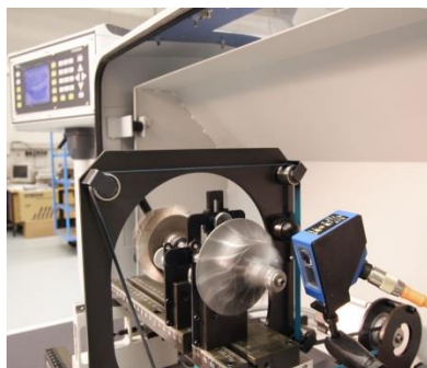
Wyważarka Schenck
